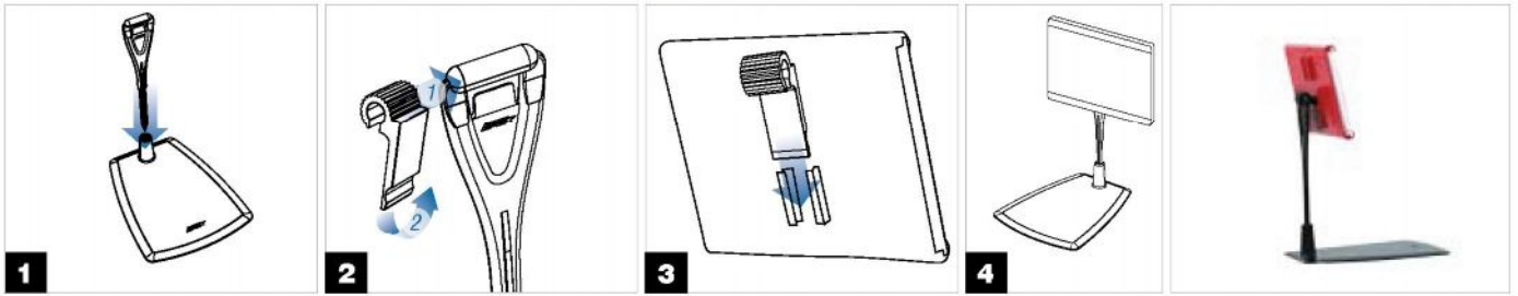
Установка на подставке с помощью DELI-STICK
