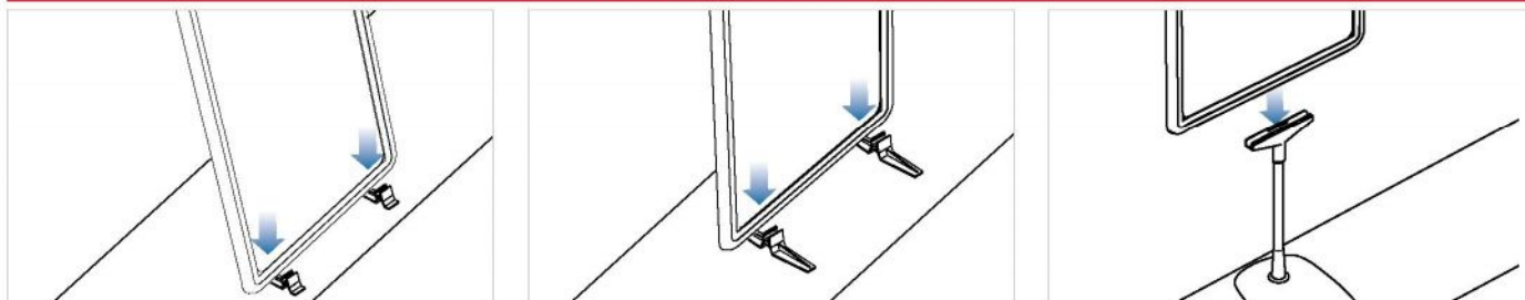
Установка пластиковых рамок на горизонтальных плоскостях
